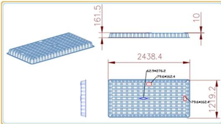
Bandejas 4'x8'x6 "
